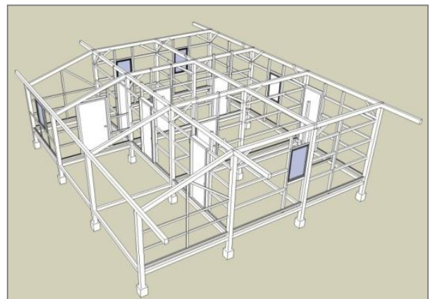
Gambar 7: Rangka Bangunan Rumah Tradisional Pulo
