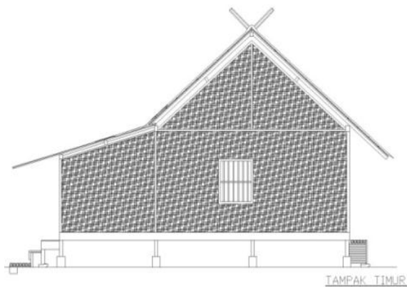
Gambar 4: Tampak Samping Rumah Tradisional Pulo
