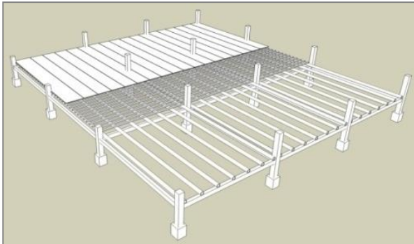
Gambar 6: Bentuk Rangka Lantai Rumah Tradisional Pulo
