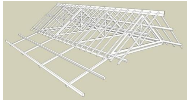
Gambar 8: Bentuk Rangka Kuda-kuda Atap Rumah Tradisional Pulo
