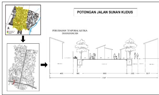
Gambar 13. Perubahan Fungsi & Dimensi Jalan (Analisa Peneliti, 2019)
