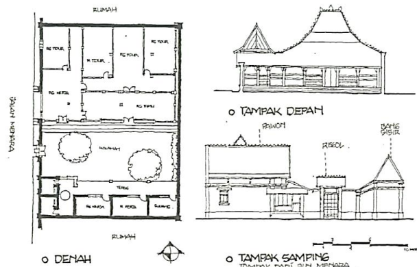
Gambar 2. Rumah Tradisional Pencil Kudus (Sardjono B. A., 2009)
